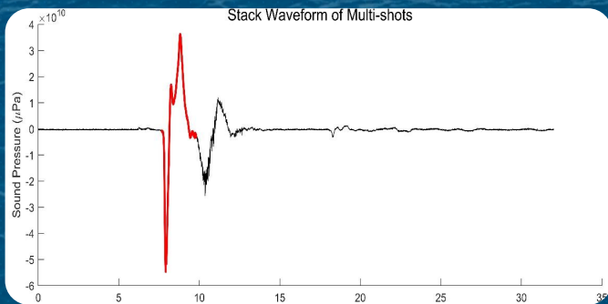
波形测试 e-Sparker 200 @1000J
